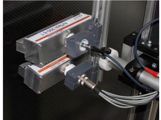
Bild 2: Einseitige Prüfung mit V-Anordnung der Arrays
