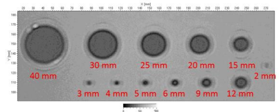
Bild 4: Auflösung von Flachbodenbohrungen in 5,3 mm dickem CFK mit 300 kHz Prüffrequenz
