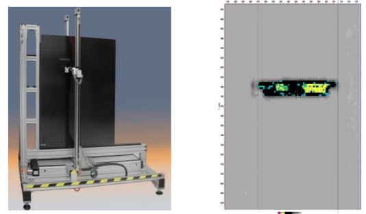
Bild 5: Prüfung einer CFK-Platte im FlatScan 1000, simulierte Fehlstelle wird im C-Bild angezeigt
